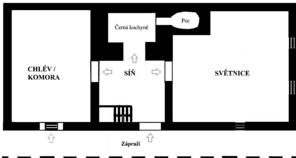
Půdorys domu s trojdielnou dispozicí - základní budova polabských usedlostí (nejen) 16. století
